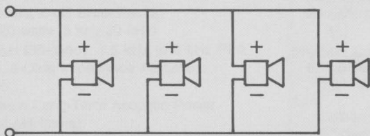
2-OHM LOAD
