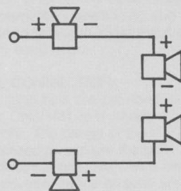
32-OHM LOAD
